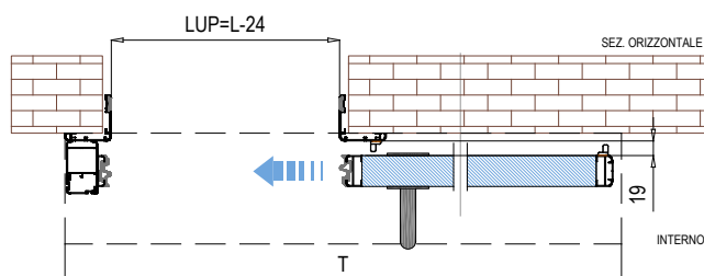
1 ANTA SCORREVOLE CON CORNICE SEMPLICE
