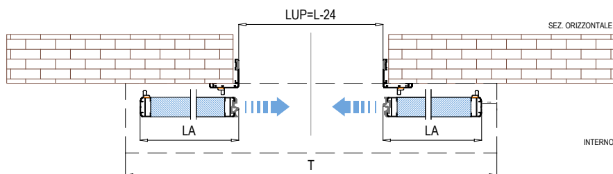
2 ANTE SCORREVOLE CON CORNICE SEMPLICE
