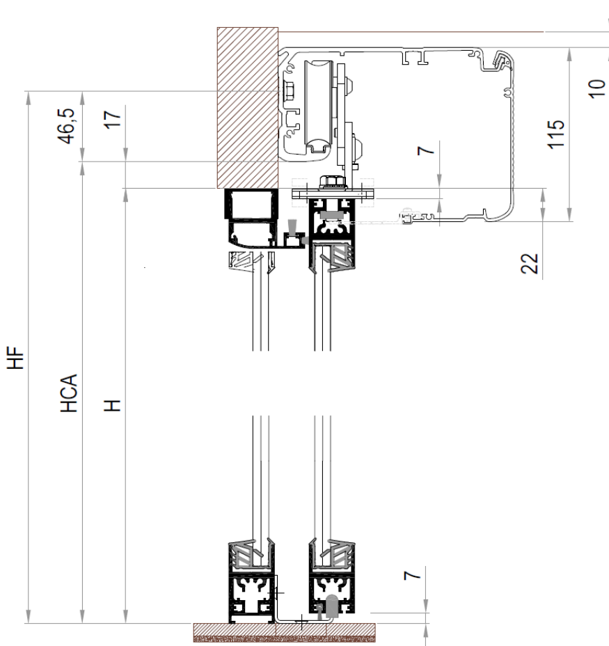
Fig.5 – S30 con hoja fija
