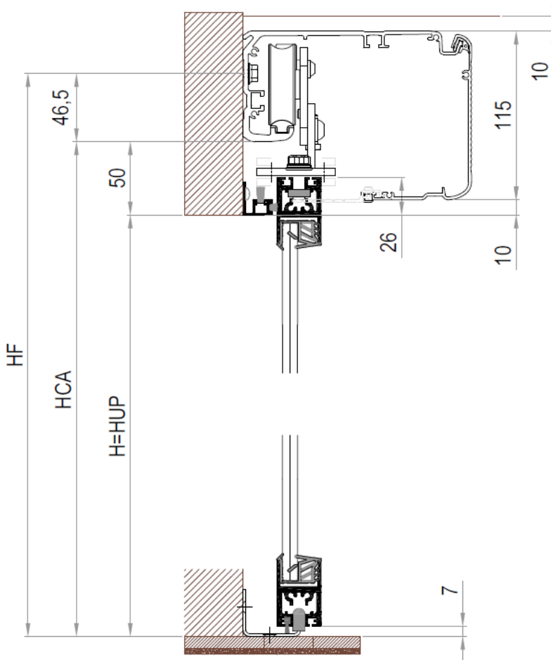
Fig.7 – Solo hoja móvil Magnum
