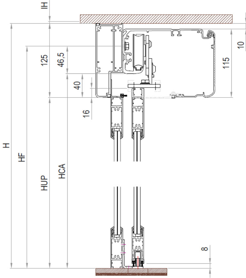
Fig.5 – S30 con hoja fija
