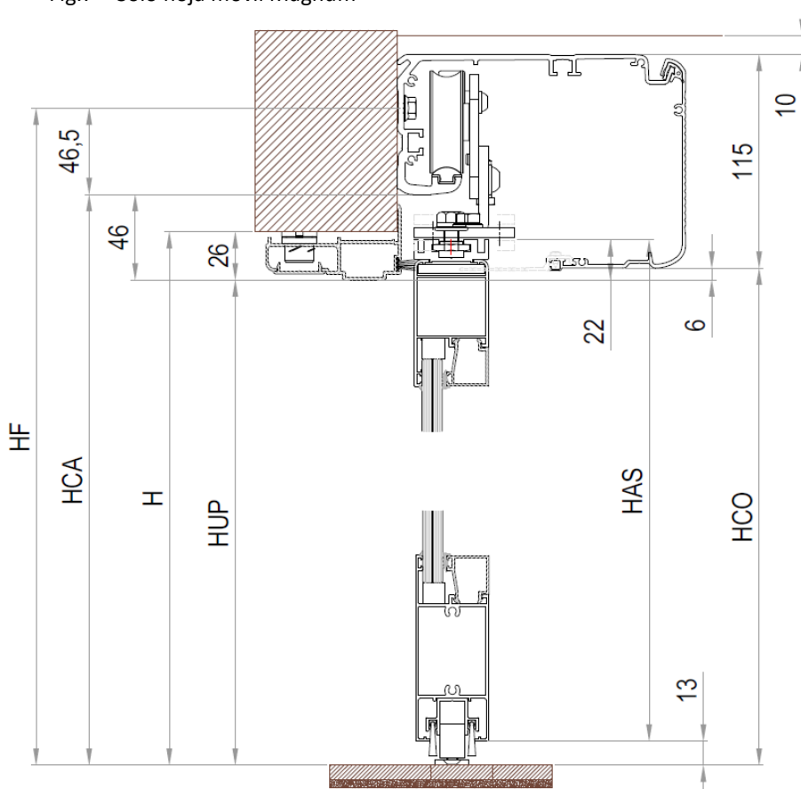
Fig.7 – Solo hoja móvil Magnum
