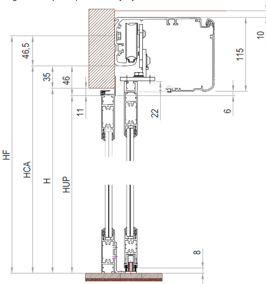
Fig.3 – Twenty en la pared con hoja fija
