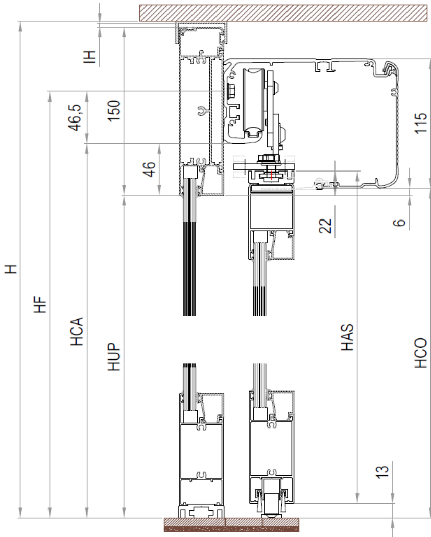
Fig.8 - Magnum con viga y hoja fija
