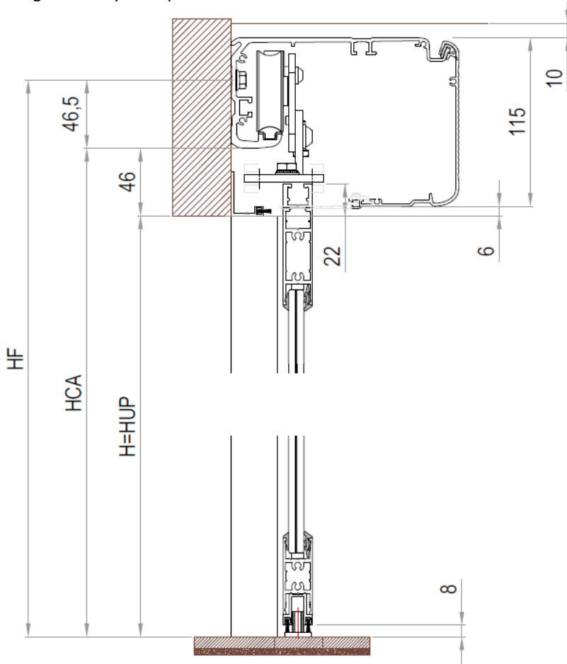
Fig.3 – Twenty en la pared con hoja fija
