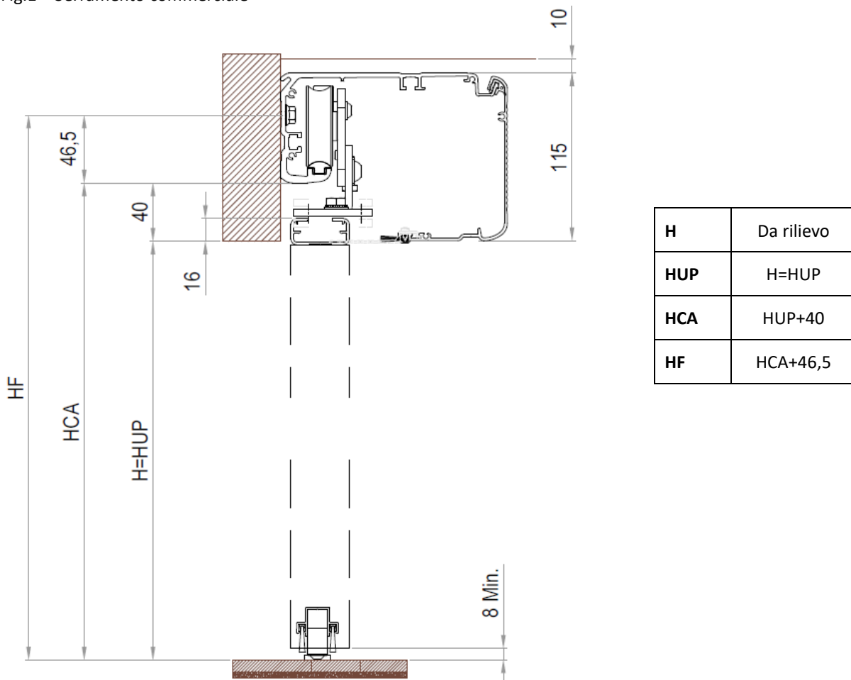
Fig.1 – Serramento commerciale
