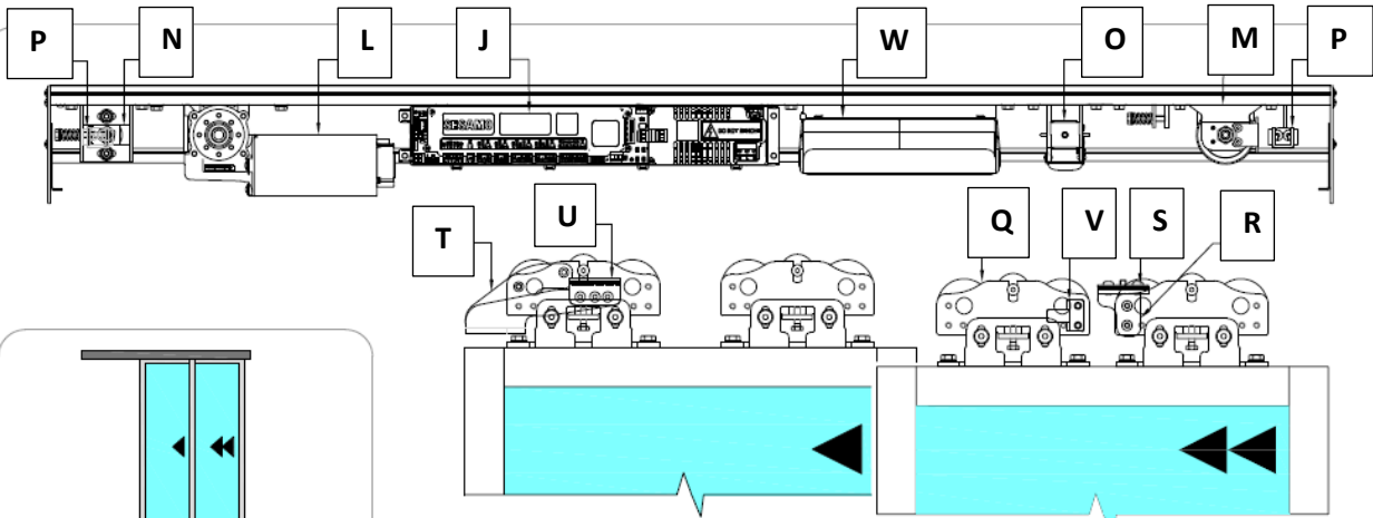
Configuration de l'entrée à 2 feuilles s'ouvre à gauche
