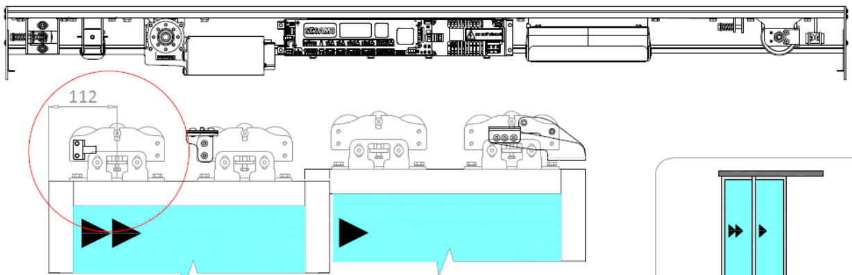
Configuration de l'entrée à deux lames s'ouvre à droite – avec électroblocs
