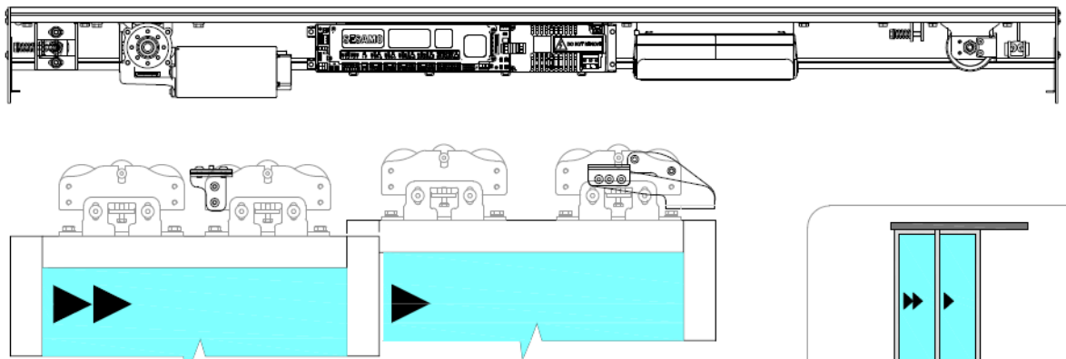
Configuration de l'entrée à deux lames s'ouvre à droite – sans électroblocs
