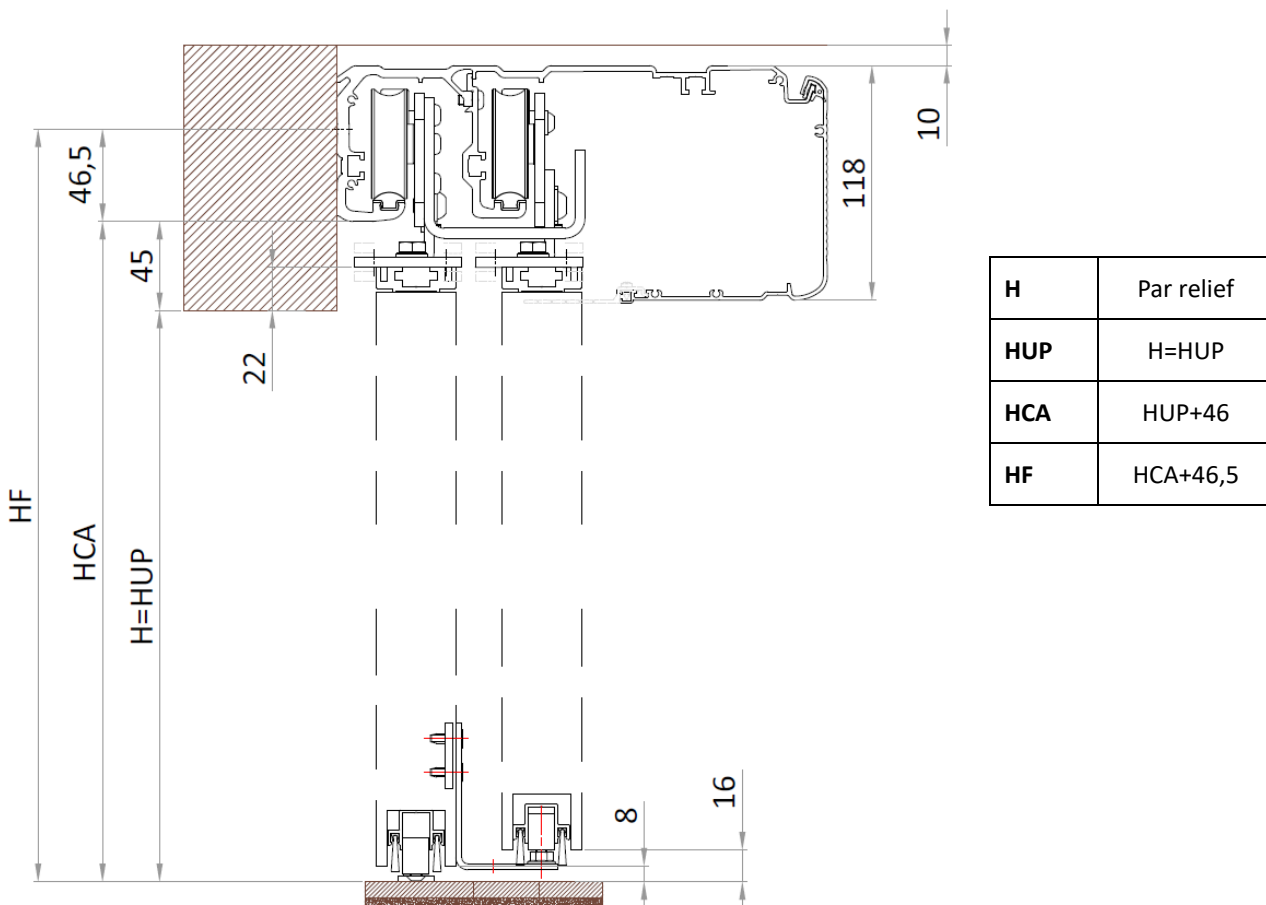
Fig.1 – Fenêtre et porte commerciales
