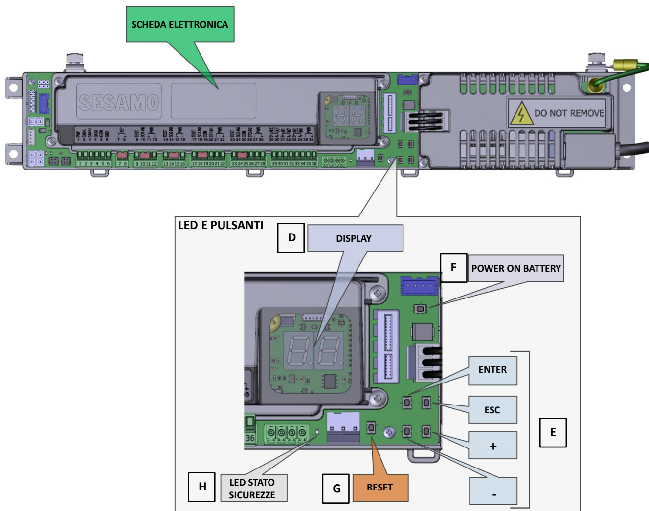
Led e Pulsanti POWERCORE
